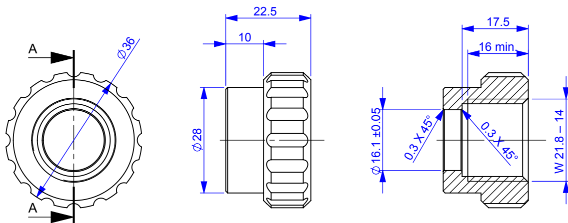
SECTION A-A
